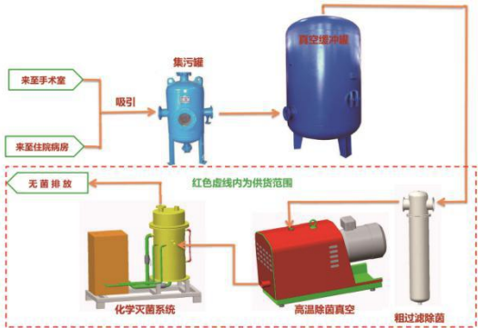
新型灭菌医院负压吸引系统流程图
