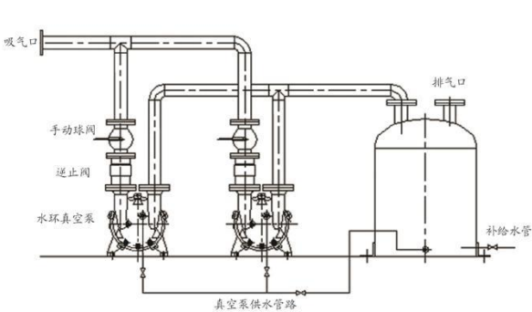
传统水环真空机组流程图
